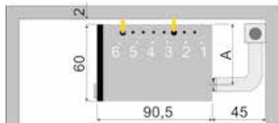
Abgasrohranschluss hinten
